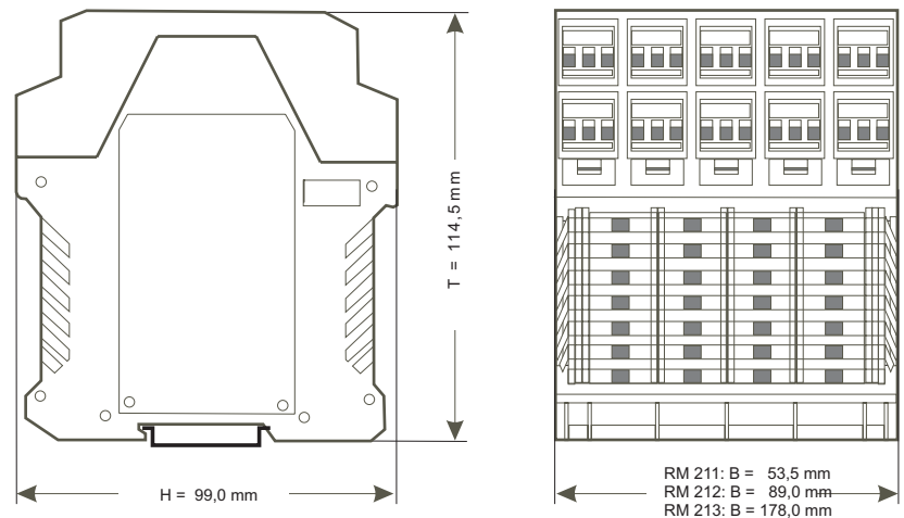
Fig. 5: Massbild RM 200 (Basismodule; dargestellt: 5-fach Basismodul RM 212)
