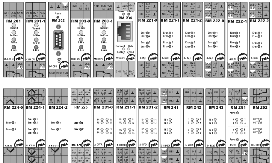
Fig. 3 : Anzeigeelemente und Anschlussbilder von RM 200-Modulen
