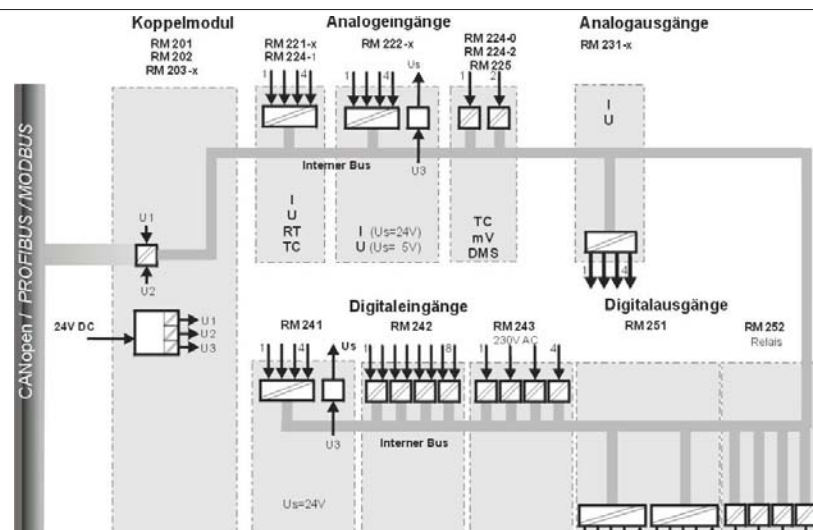
Fig.4 : Galvanische Trennungen im System
