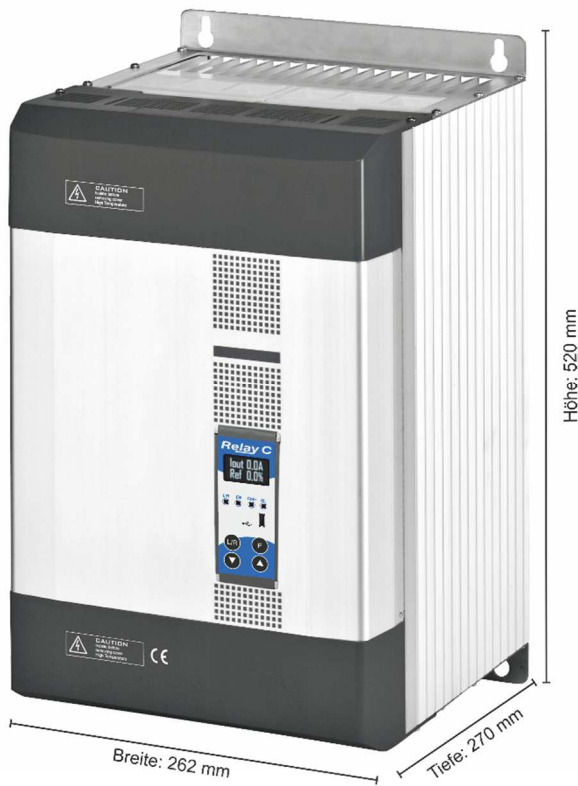
Relay C 2PH 300A...700A (S14) Gewicht 22,5 kg
