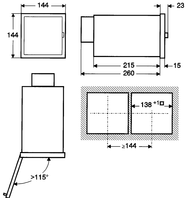
Abb. 1 Maßbild
