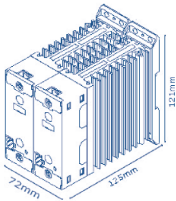
W 72 mm. - H 121 mm. - D 125 mm. - kg. 0,88 Relay S, No fuse 30A ÷ 40A
