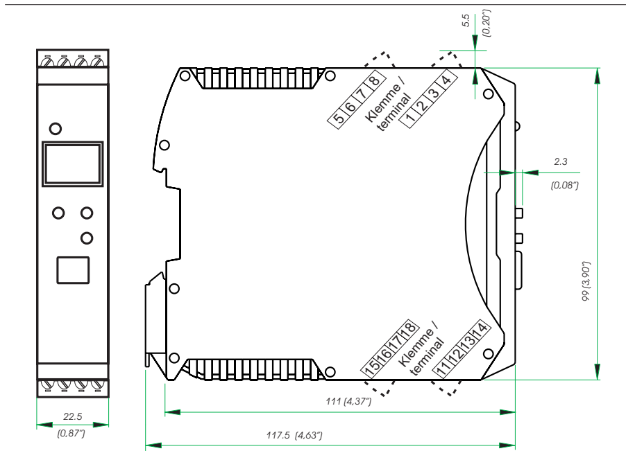
Fig. 4: Dimensions
