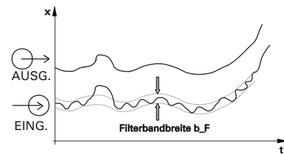
Fig. 3 : Filter function
